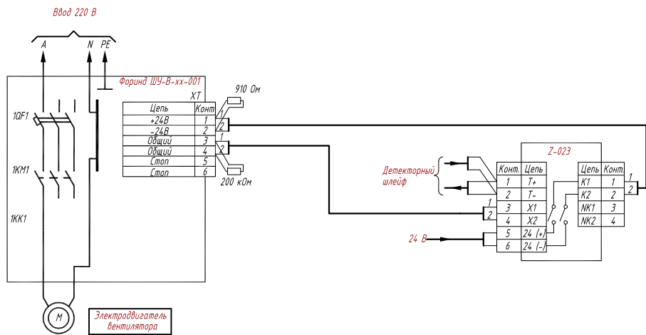
Схема подключения шкафа управления вентилятором ШУ-В-ххА-001 к сети 220В.
